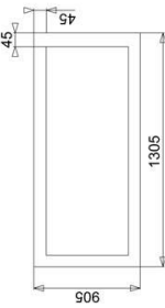
SUPERFICIE APOGGIO A PAVIMENTO FLOOR SUPPORT AREA
